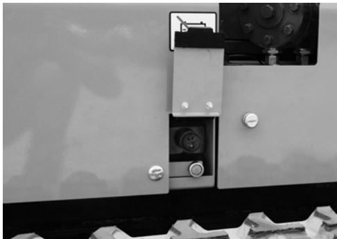
Fig. 167 Positie connector optionele tweede afstandsbediening
