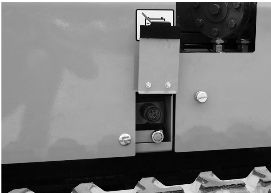
Fig. 65 Positie connector optionele tweede afstandsbediening
