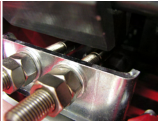
Fig. 187 Kabelschoen met zitting voor rotatieblokkende spie
