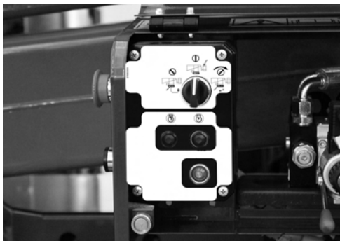
Fig. 73 Keuzeschakelaar versie met thermische motor
